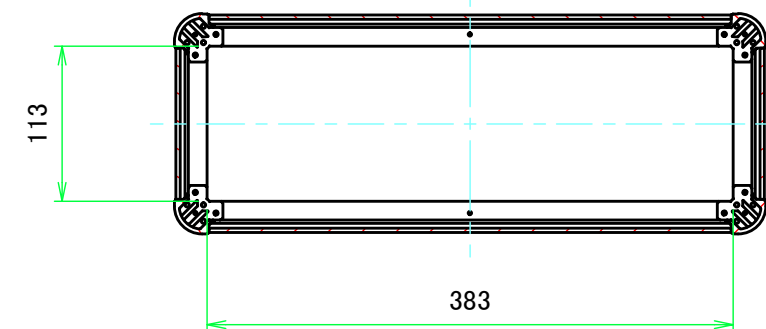
C-C (1 : 5.5)
